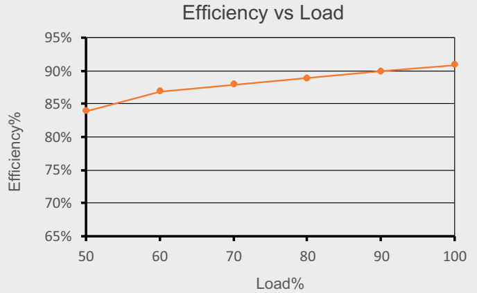
GDS-PS6024-IP68
