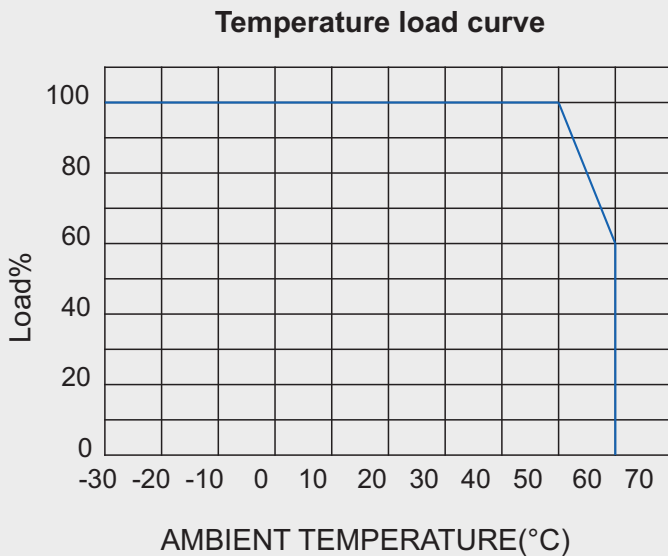
GDS-PS6012-IP68
